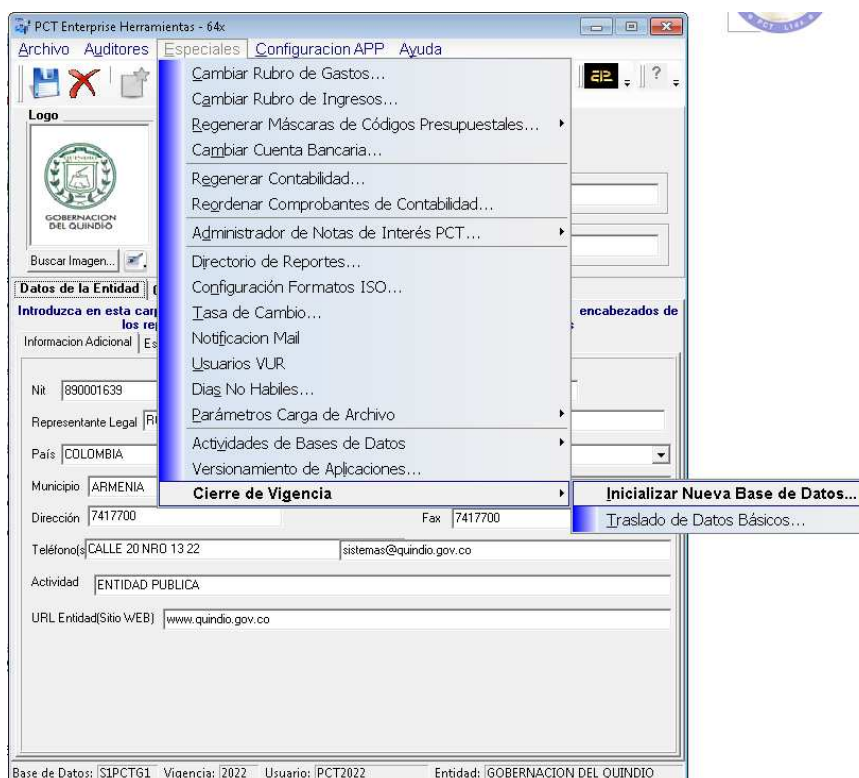
Figura 3. Menú – Inicializar Base de Datos
